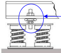
Montaje con nivelación Sistema con base superior
